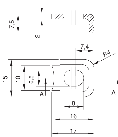
A-A KESİTİ
